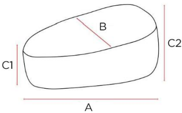
Hovedstøttepude, asymmetrisk: 0319-7201-000 A Længde 35 cm B Bredde 24 cm Højde C1 5,5 cm, C2 13 cm
