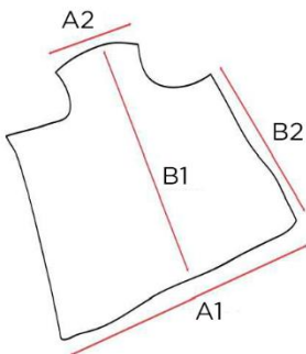
Benafslapperen (barn): 0319-7621-000 A1 Længde 60 cm, A2 Længde 20 cm B1 Bredde 100 cm, B2 Bredde 81 cm
