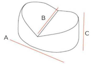
Hovedstøttepude, symmetrisk: 0319-7211-000 A Længde 35 cm B Bredde 24 cm C Højde 13 cm
